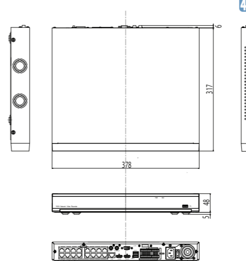
裏面図
