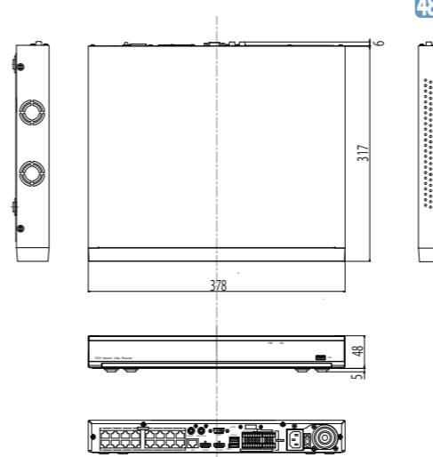
裏面図
