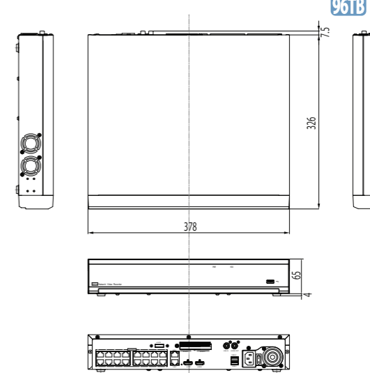
裏面図
