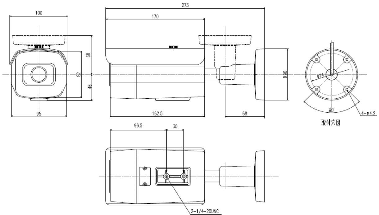
外形寸法図
