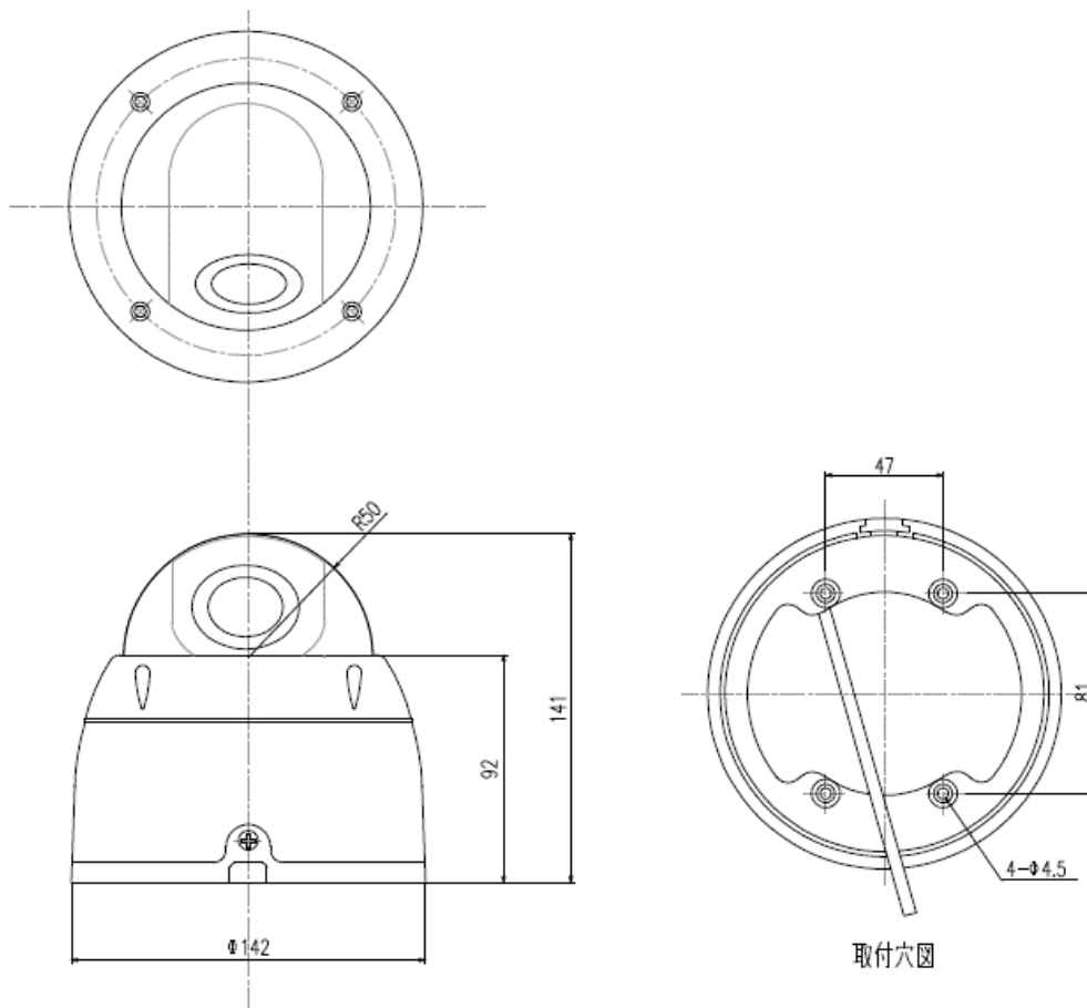
外形寸法図
