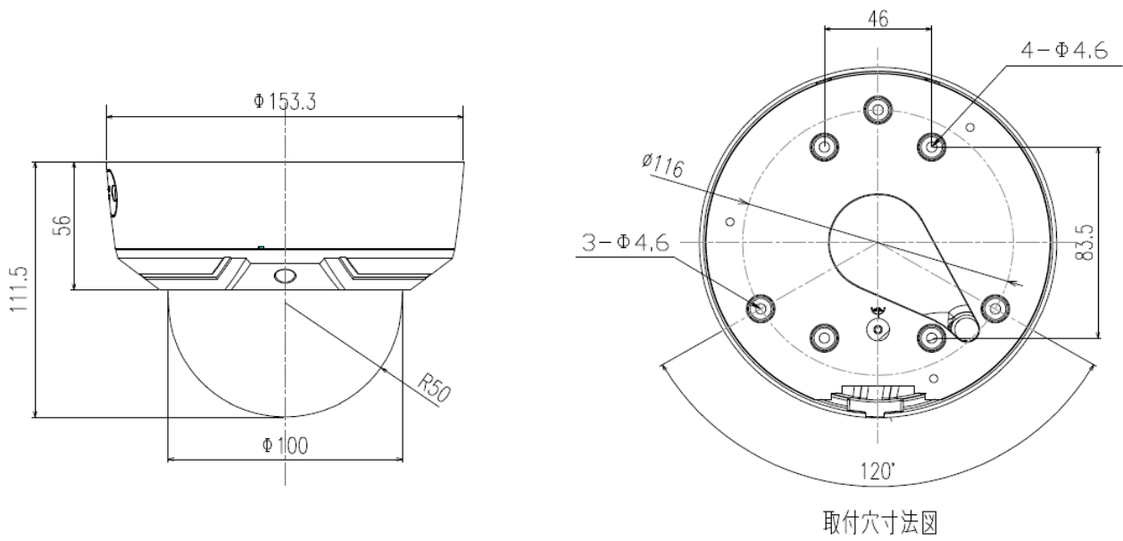
TNC-3203 外観図
