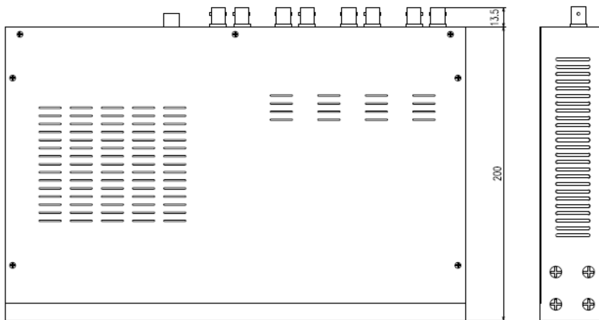
外形寸法図
