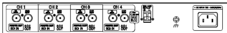
裏面図
