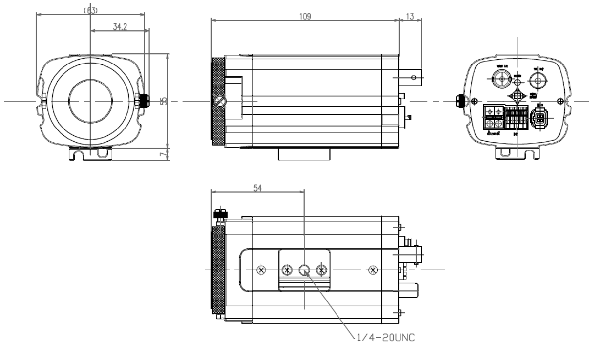
外形寸法図
