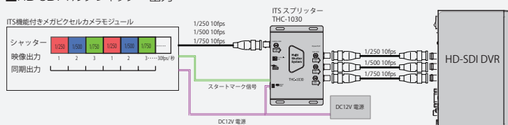
シャッター1(低速) シャッター2(中速) シャッター3(高速)
